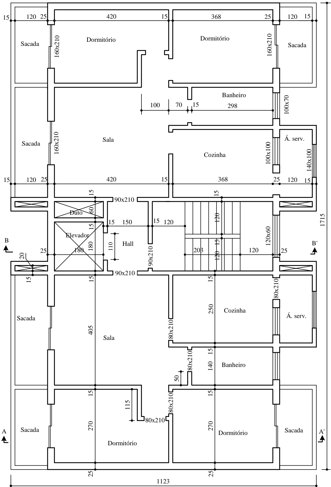
Planta baixa do pavimento tipo
