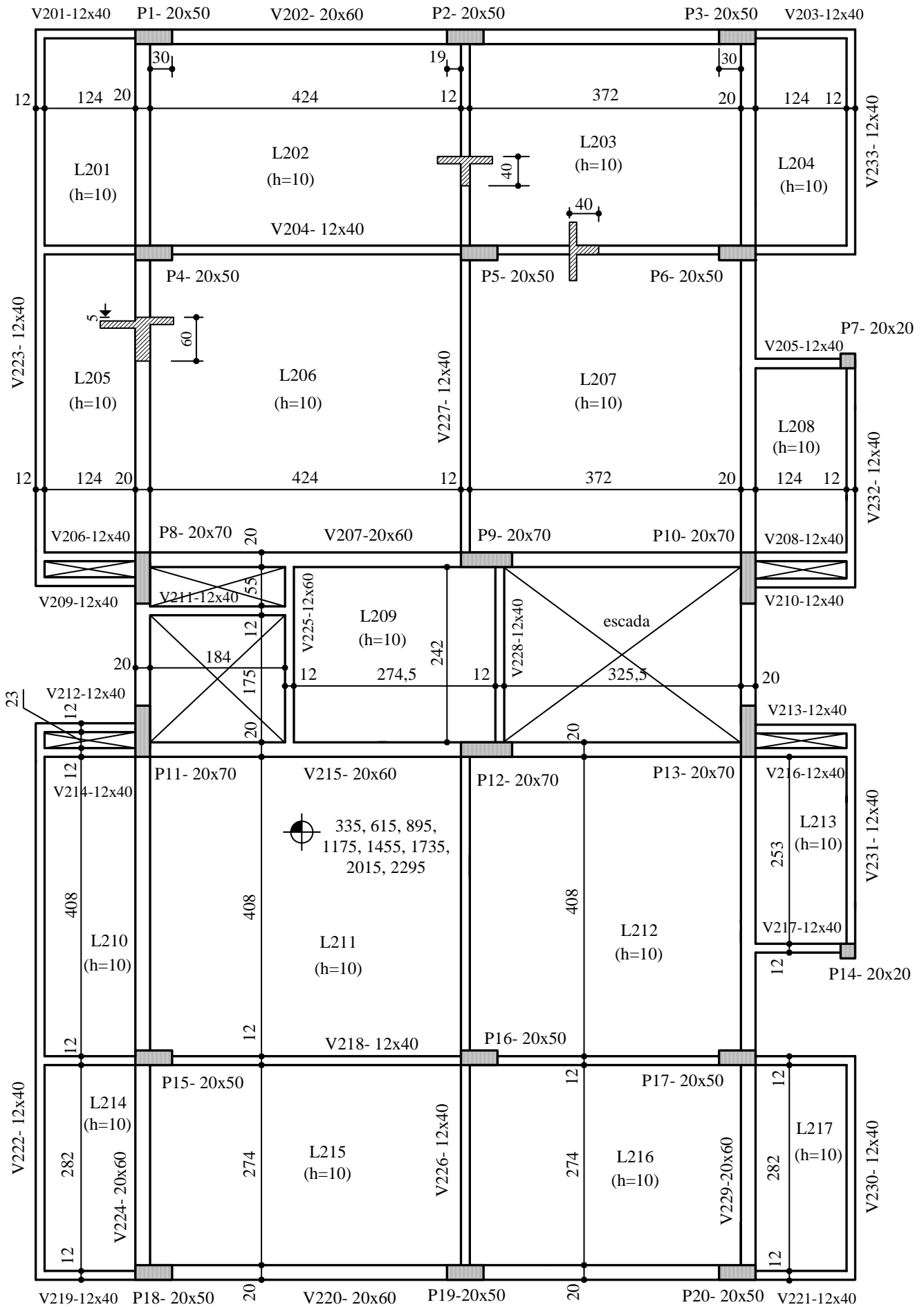
Formas do pavimento tipo
